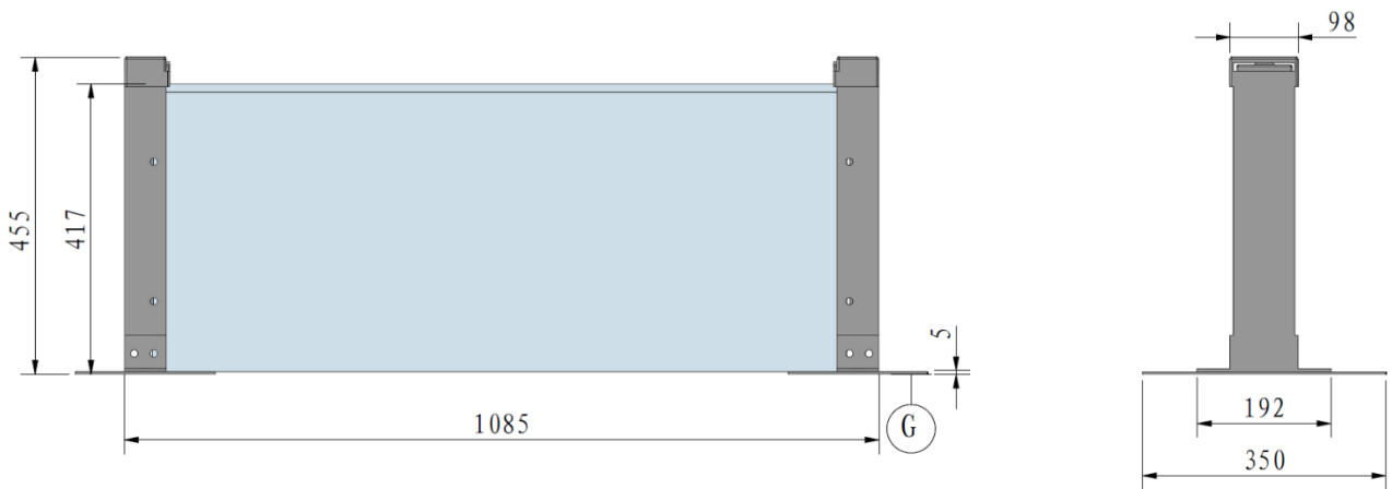
图 3-15 掩体示意图
