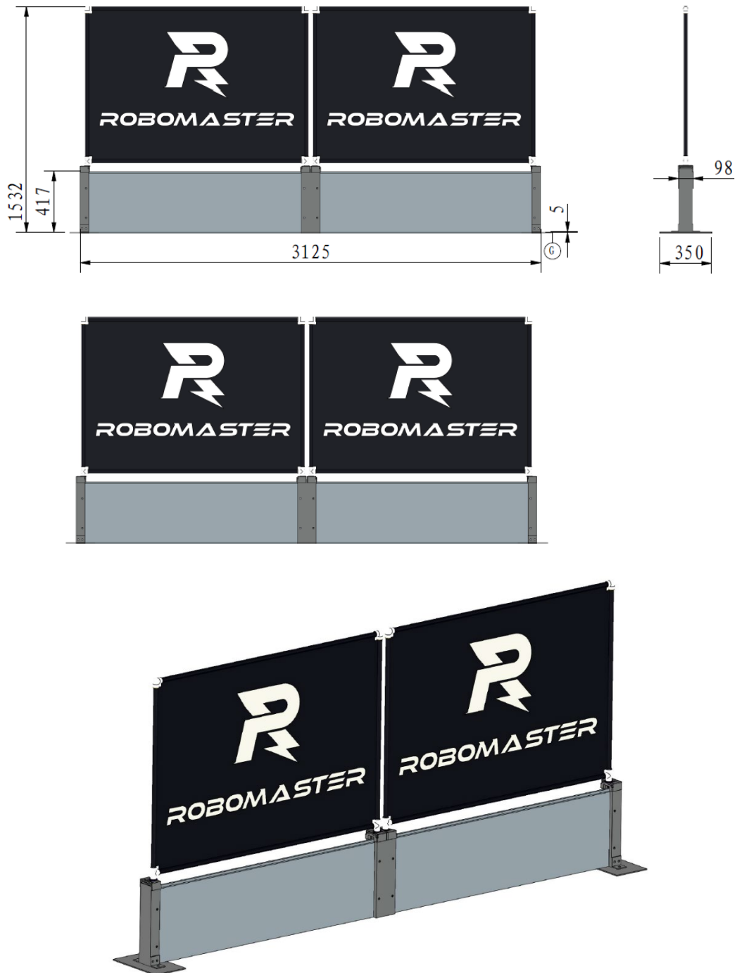
图 3-10 掩体示意图
